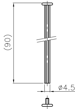
組ネジ
